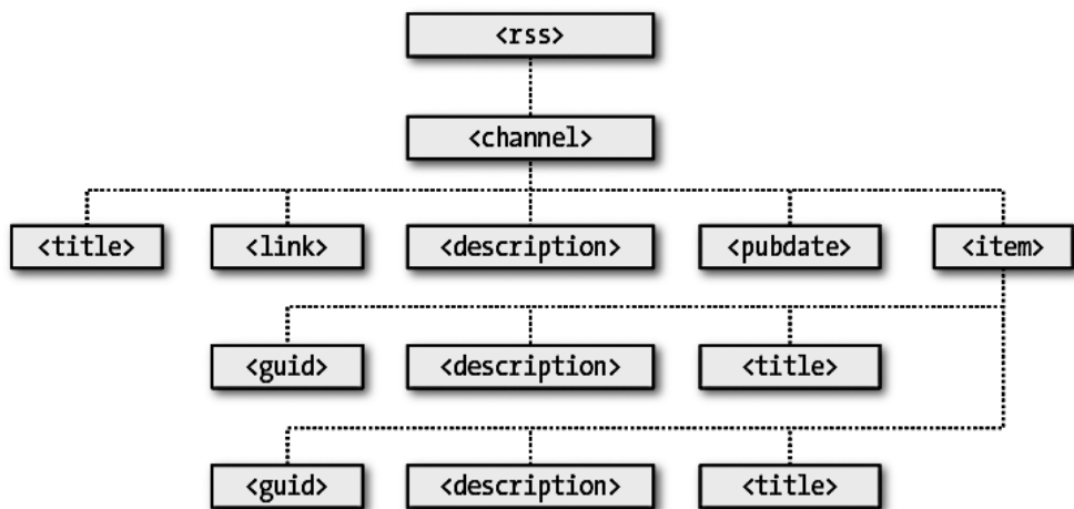
Рис. 17.3. DOM-дерево примера 17.8
